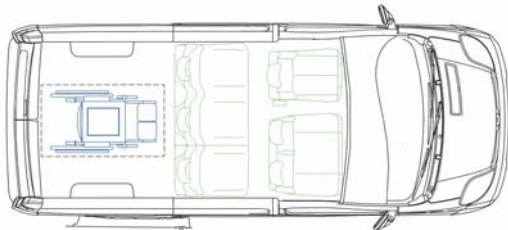
C1 – 5/6 places + 1 fauteuil roulant
