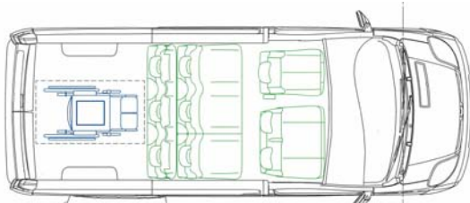
L2H1 - 5/6 places + 1 fauteuil roulant
