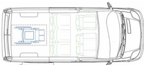
L1H1 - 5/6 places + 1 fauteuil roulant
